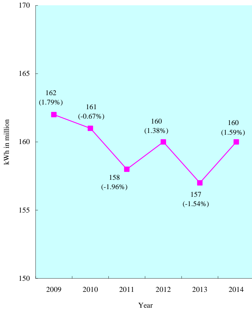
圖1：2009-2014年電力耗用量 Figure 1 : Electricity Consumption 2009-2014 Calendar Year
